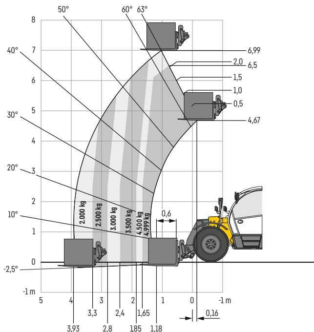
T 55-7s mit Pendelachssperre
